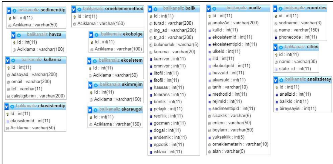
Şekil 1. Veri Tabanı Ekran Görüntüsü
