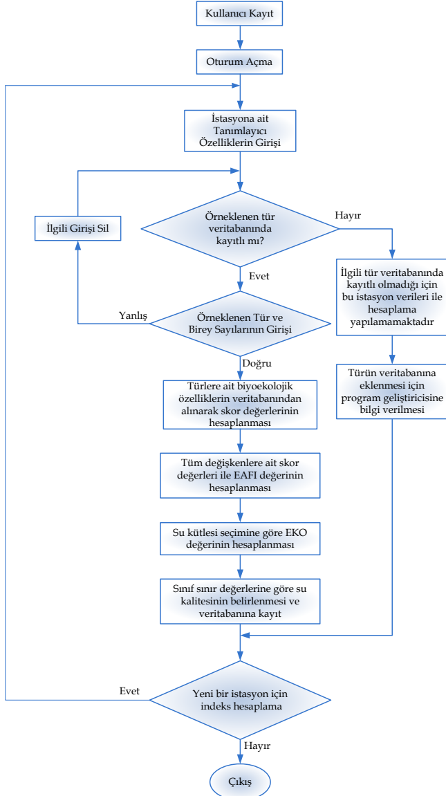
Şekil 6. İndeks Verilerinin Temel Giriş Algoritması
